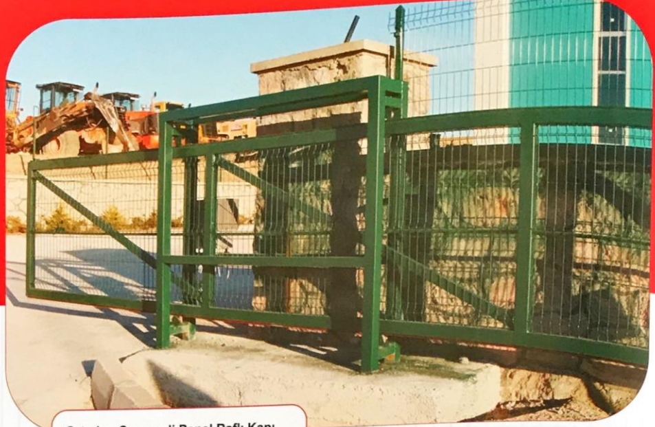
Ortadan Çerçevesiz Panel Rafı Kapı 50 x 150 x 4.5 x 5 mm
